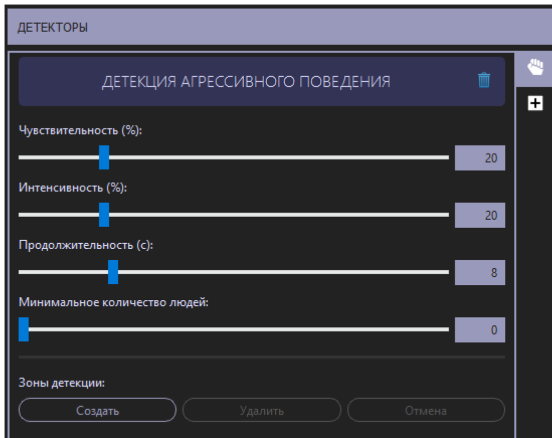
Рисунок 35. Настройка детектора «Агрессивное поведение»
