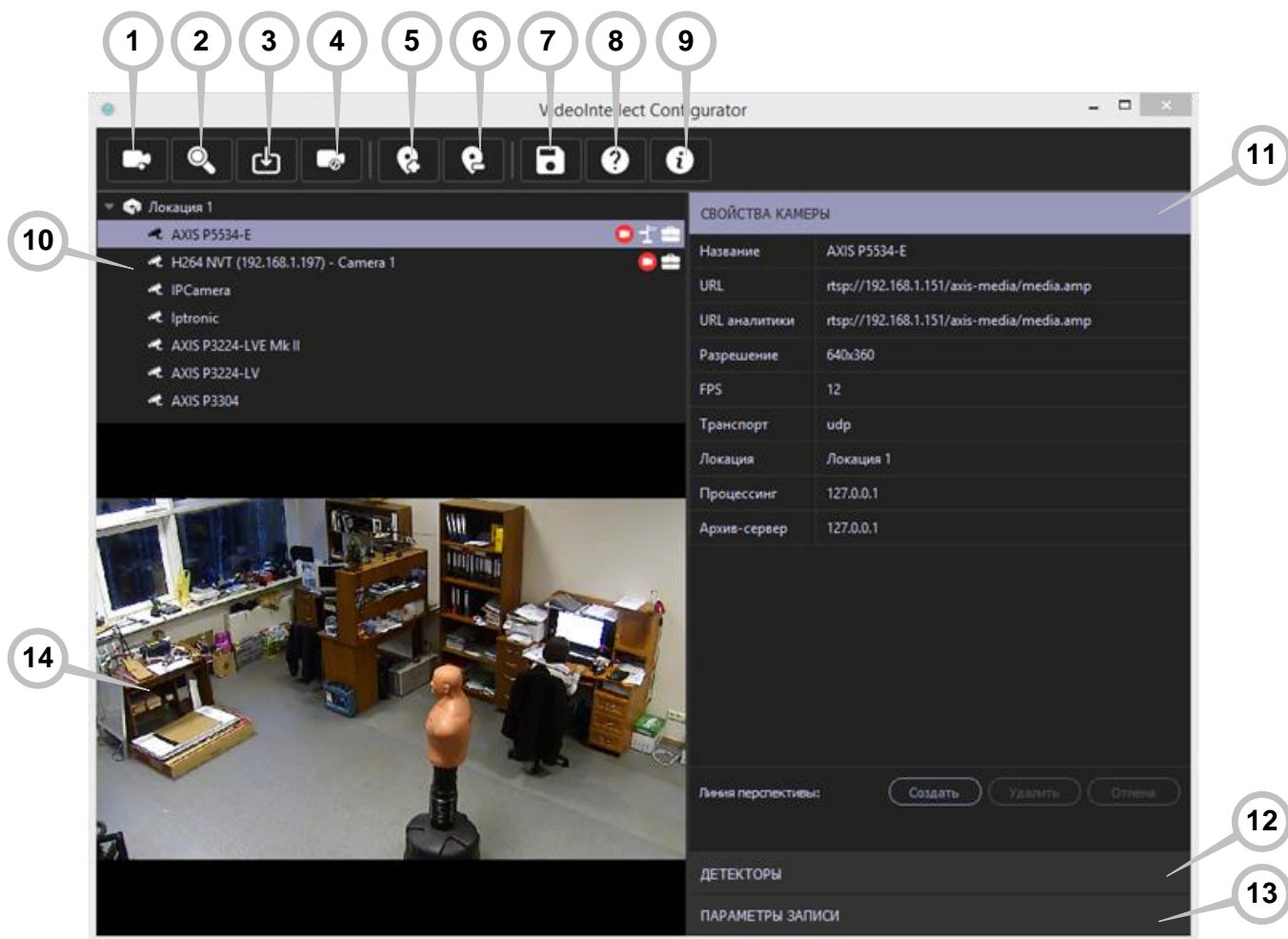
Рисунок 10. Программа «VideoIntellect-Конфигуратор». Интерфейс
