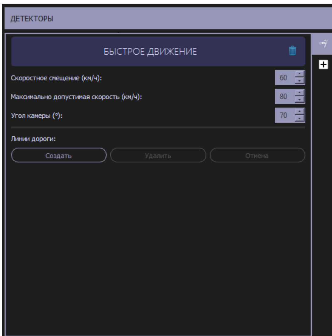
Рисунок 55. Настройка детектора «Быстрое движение»
