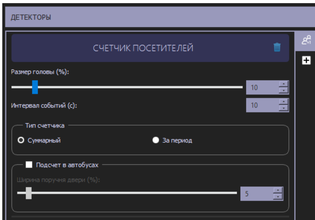
Рисунок 47. Настройка основных параметров детектора «Счетчик посетителей»
