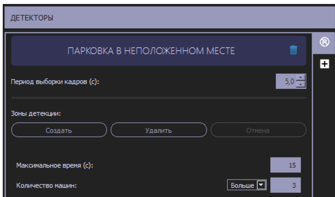
Рисунок 38. Настройка детектора «Парковка в неполюженном месте»
