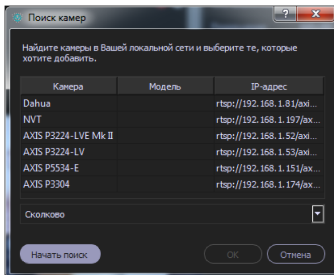
Рисунок 11. Окно «Поиск камер»
