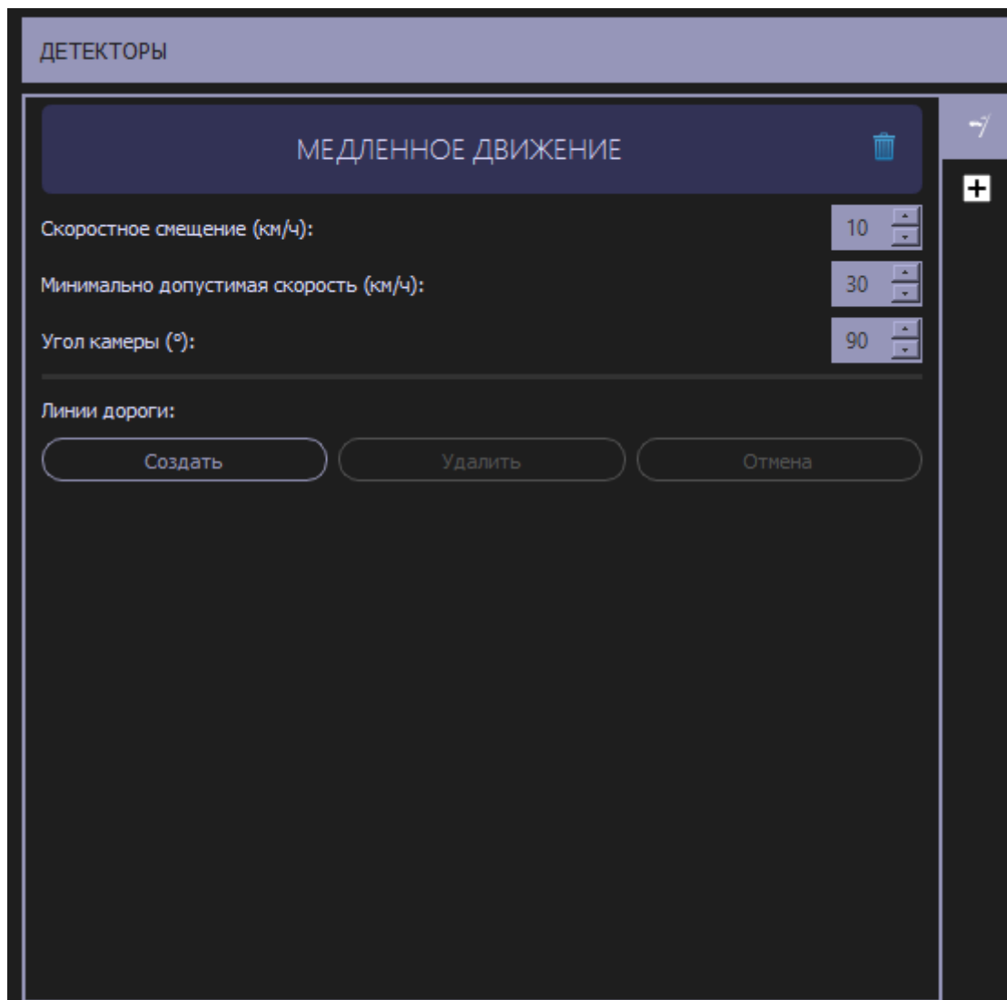
Рисунок 52. Настройка детектора «Медленное движение»
