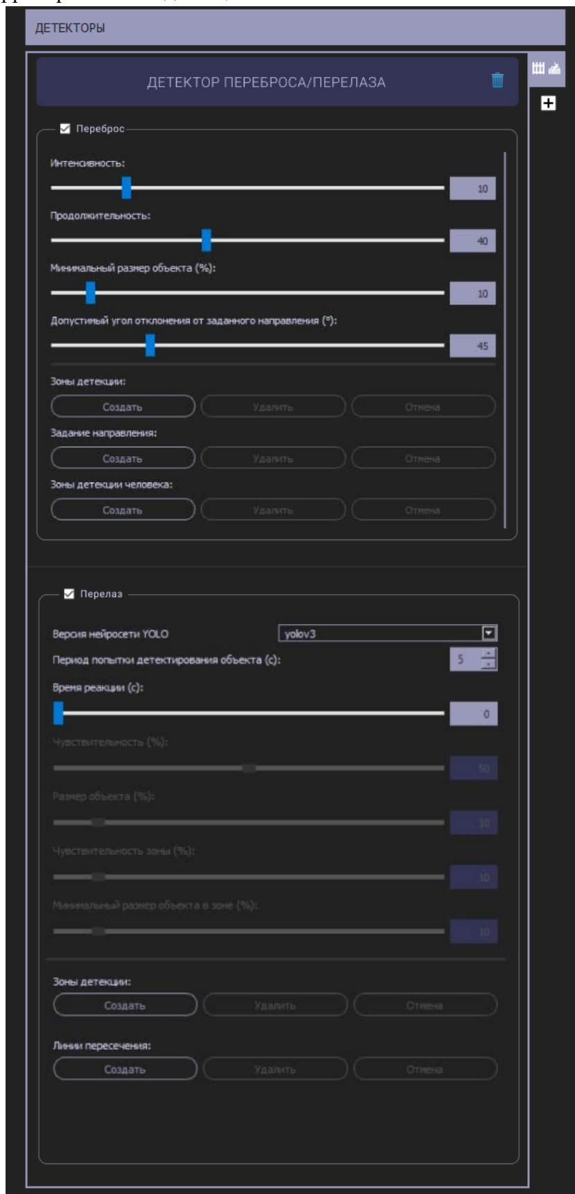
Рисунок 40. Настройка детектора «Переброс/перелаз»
