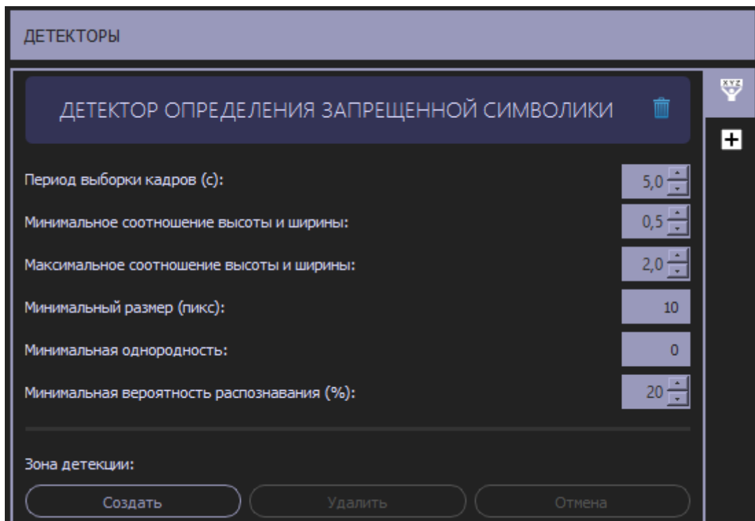
Рисунок 39. Настройка детектора «Определение запрещенной символики»
