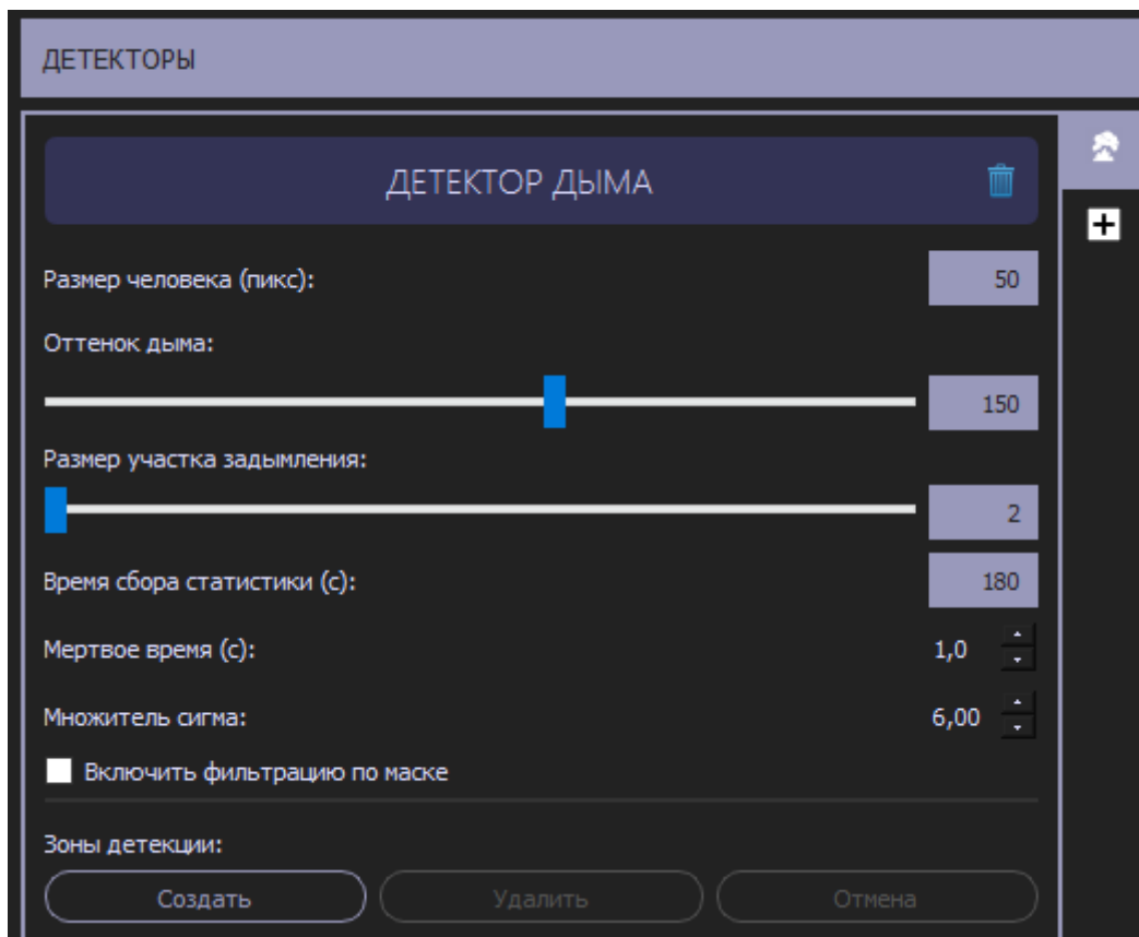
Рисунок 33. Настройка детектора «Дым»
