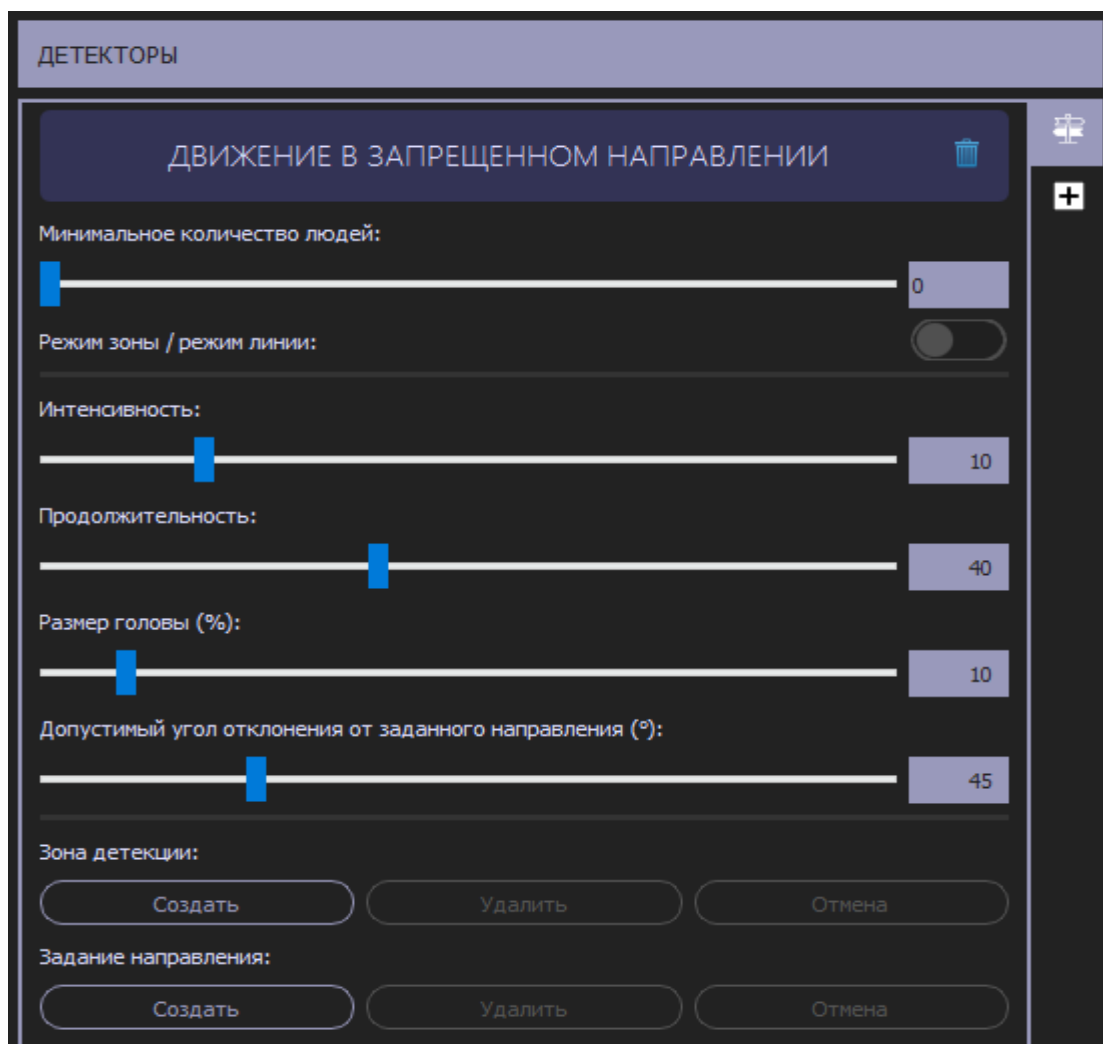
Рисунок 27. Настройка детектора «Движение в запрещенной зоне»
