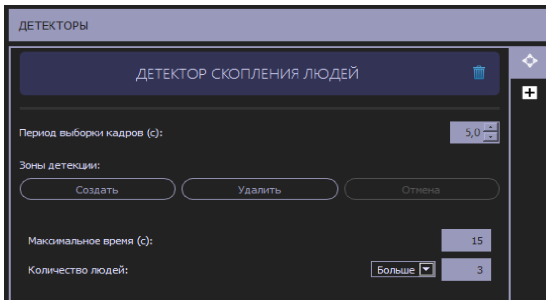
Рисунок 37. Настройка детектора «Скопление людей»
