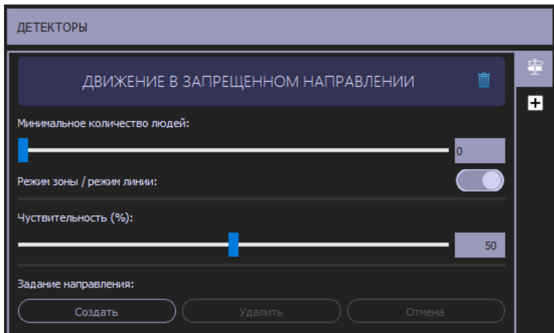
Рисунок 25. Настройка детектора «Движение в запрещенном направлении» в режиме линии
