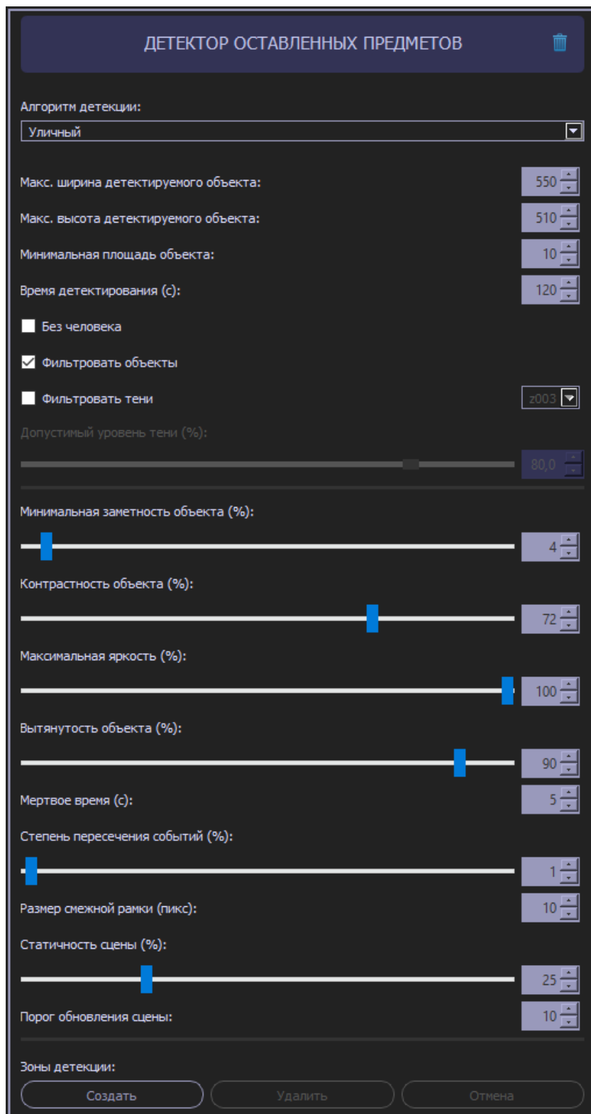
Рисунок 21.6. Панель настройки параметров детектора (режим «Уличный»)
