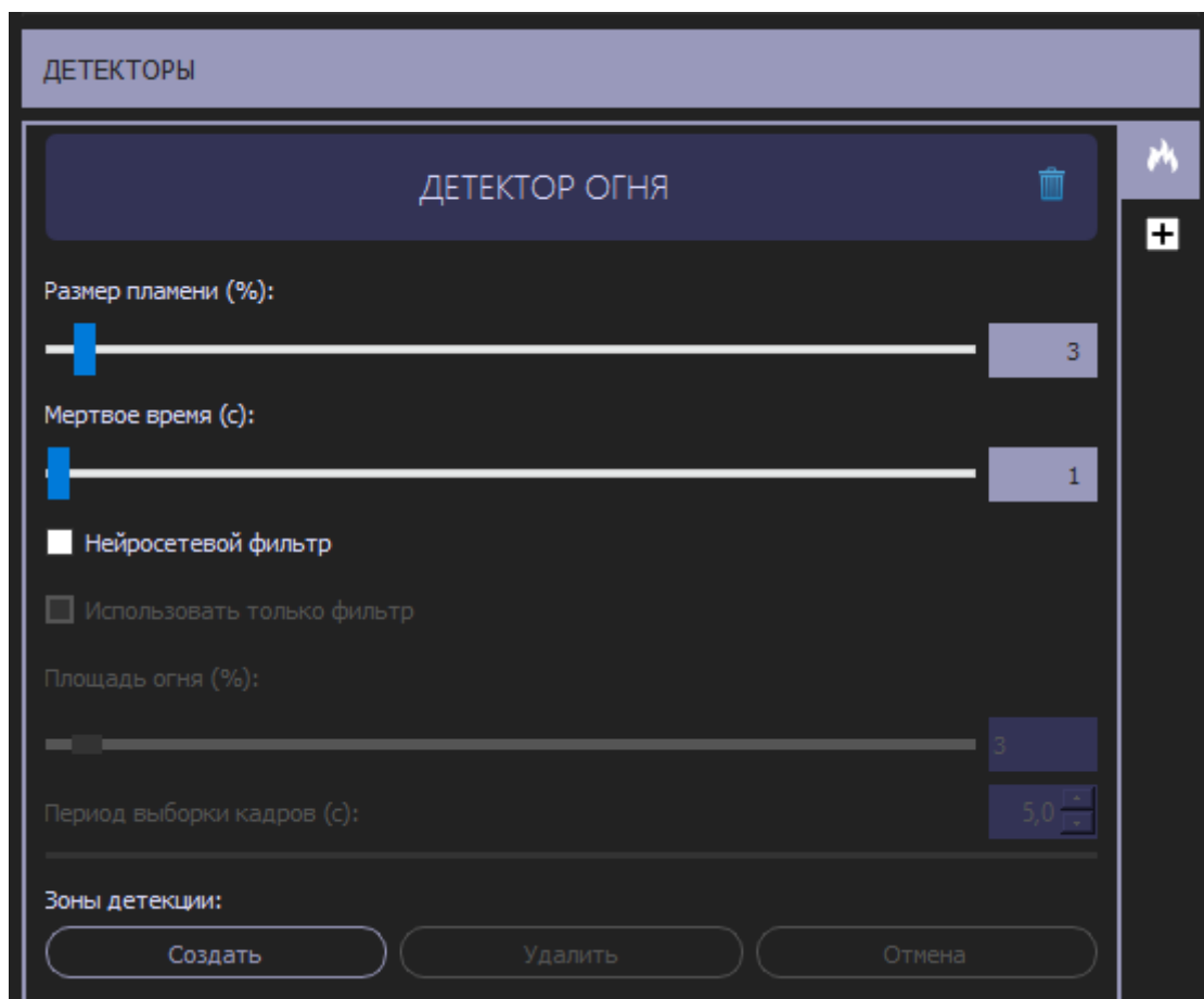
Рисунок 34. Настройка детектора «Огонь»
